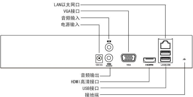
图2-2 1 盘位设备后面板示意图
