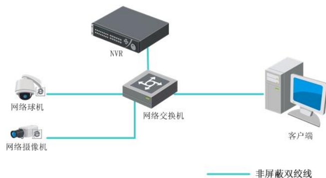
图3-1 典型应用图
