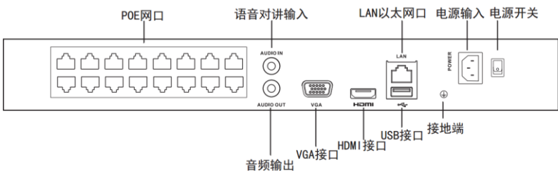
图2-5 2 盘位带 PoE 接口设备后面板示意图
