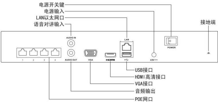
图2-4 1 盘位带 PoE 接口设备后面板示意图
