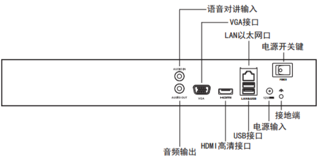
图2-3 2 盘位设备后面板示意图
